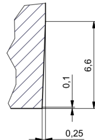
C (5 : 1)
